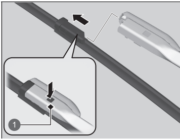
1 Lasche
