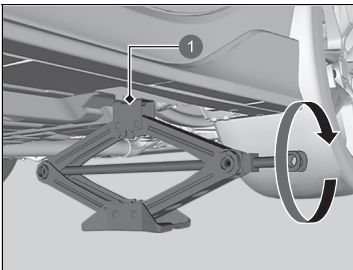
1 Hebeplatz
